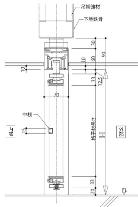
・シリンダー部 詳細図(下框タイプ)
