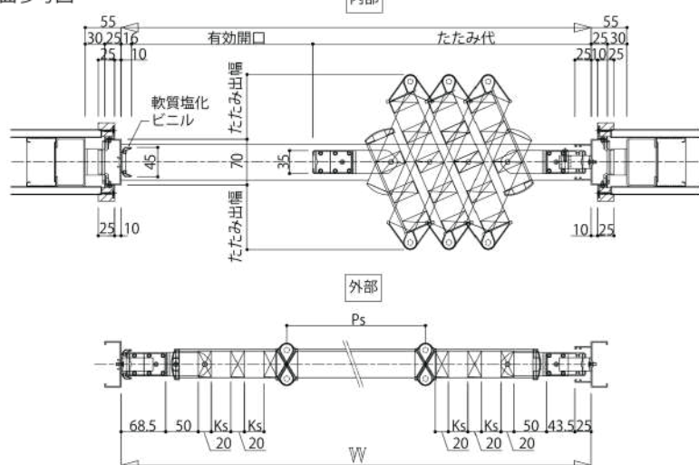
・横断面参考図
