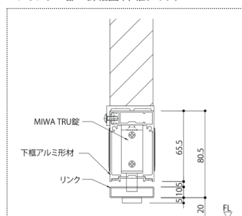
・シリンダー部 詳細図(下框タイプ)
