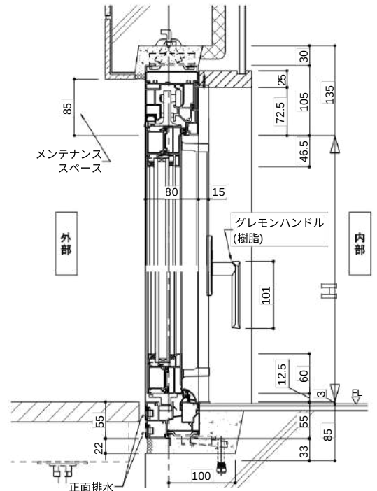
・縦断面参考図
