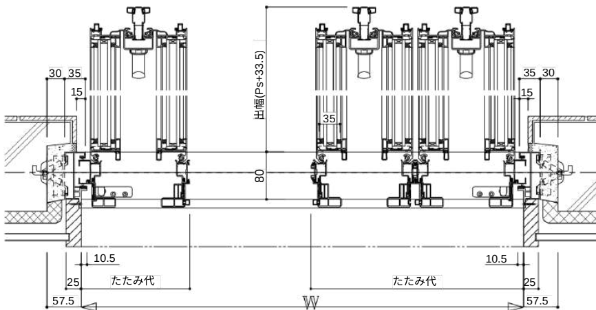
・横断面参考図
