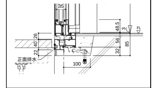
・縦断面参考図(段付き枠)DJ型
