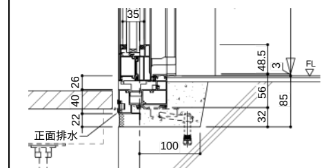
・縦断面参考図(段付き枠)DJ型
