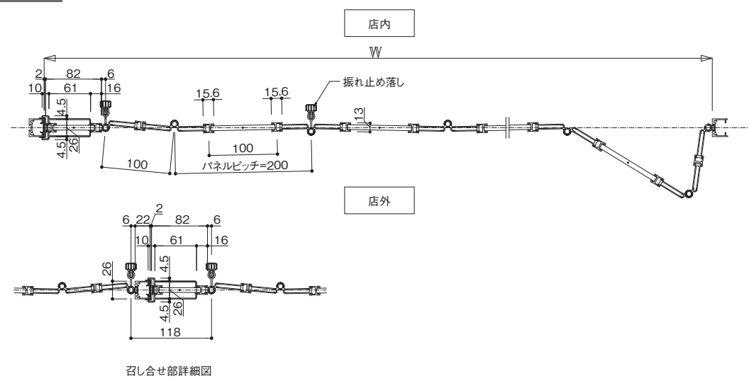
直線納まり図
