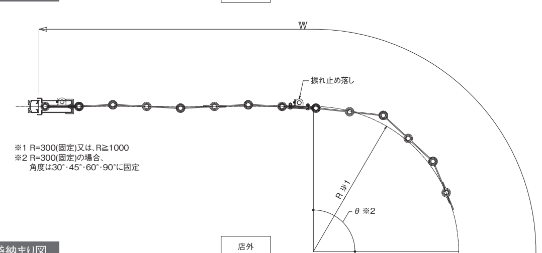
曲線納まり図
