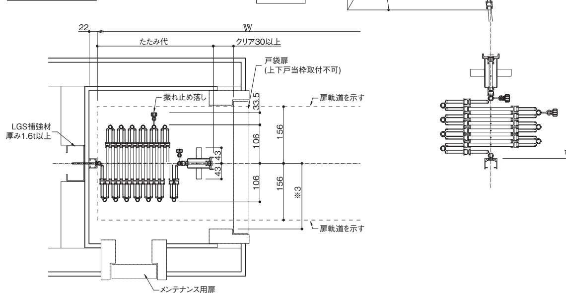
戸袋納まり図
