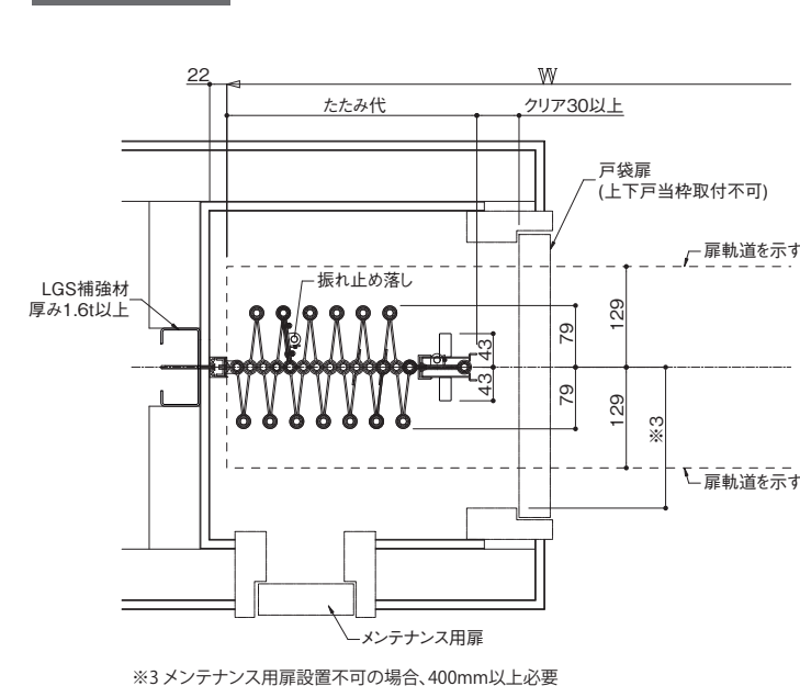
戸袋納まり図
