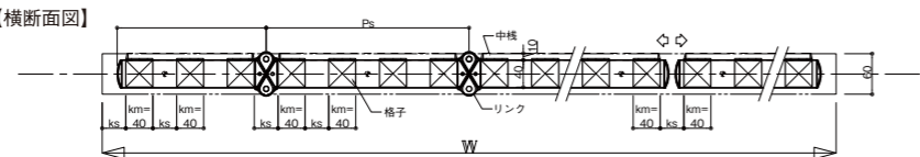
【横断面図】
