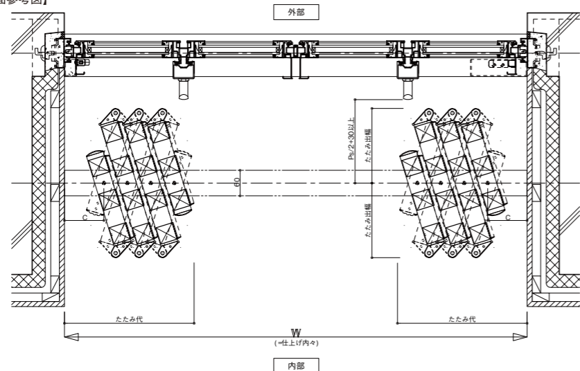
【横断面図】
