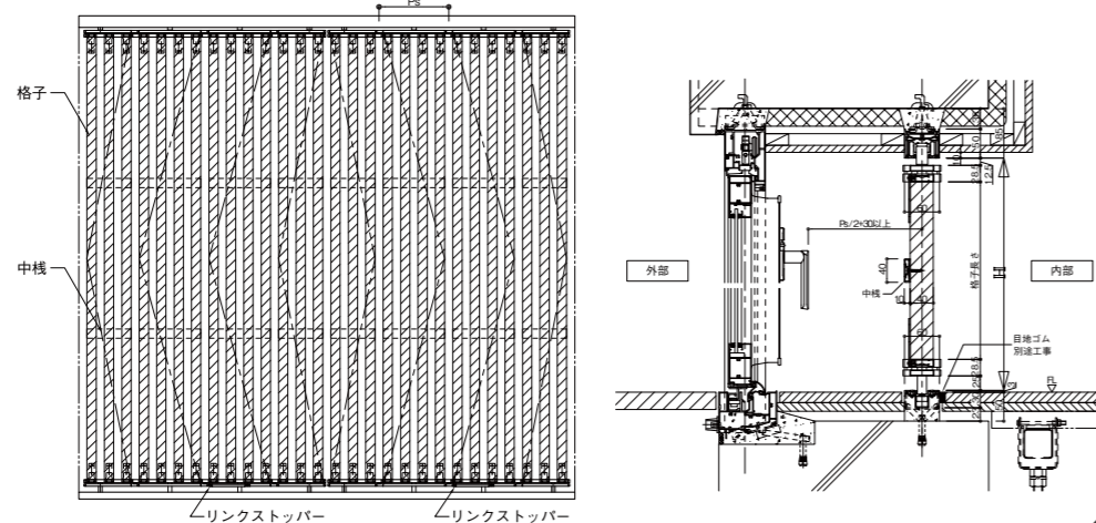
【横断面参考図】
