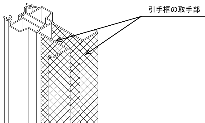
障子全閉図
