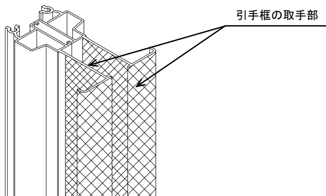
障子全閉図
