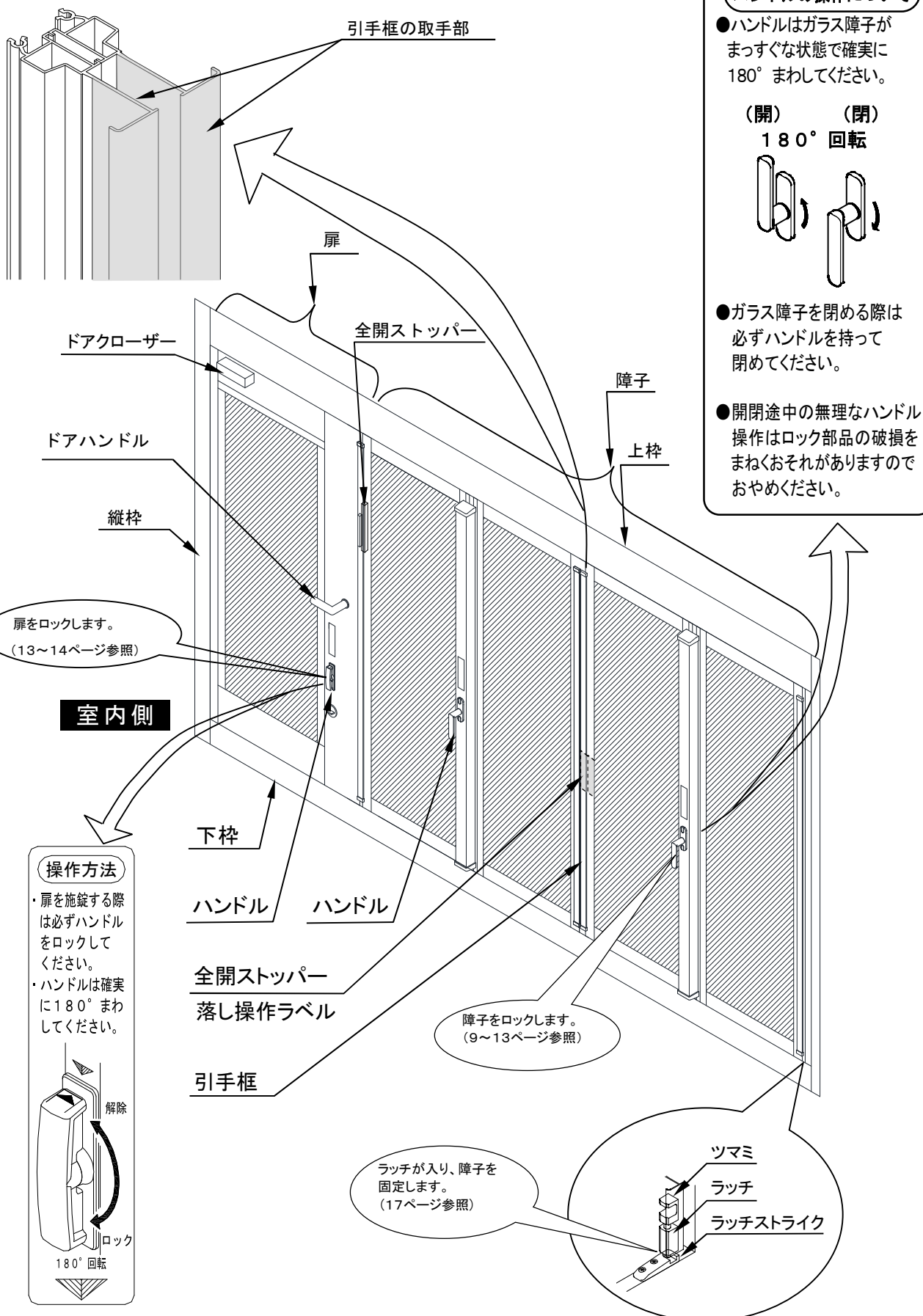
障子全閉図
